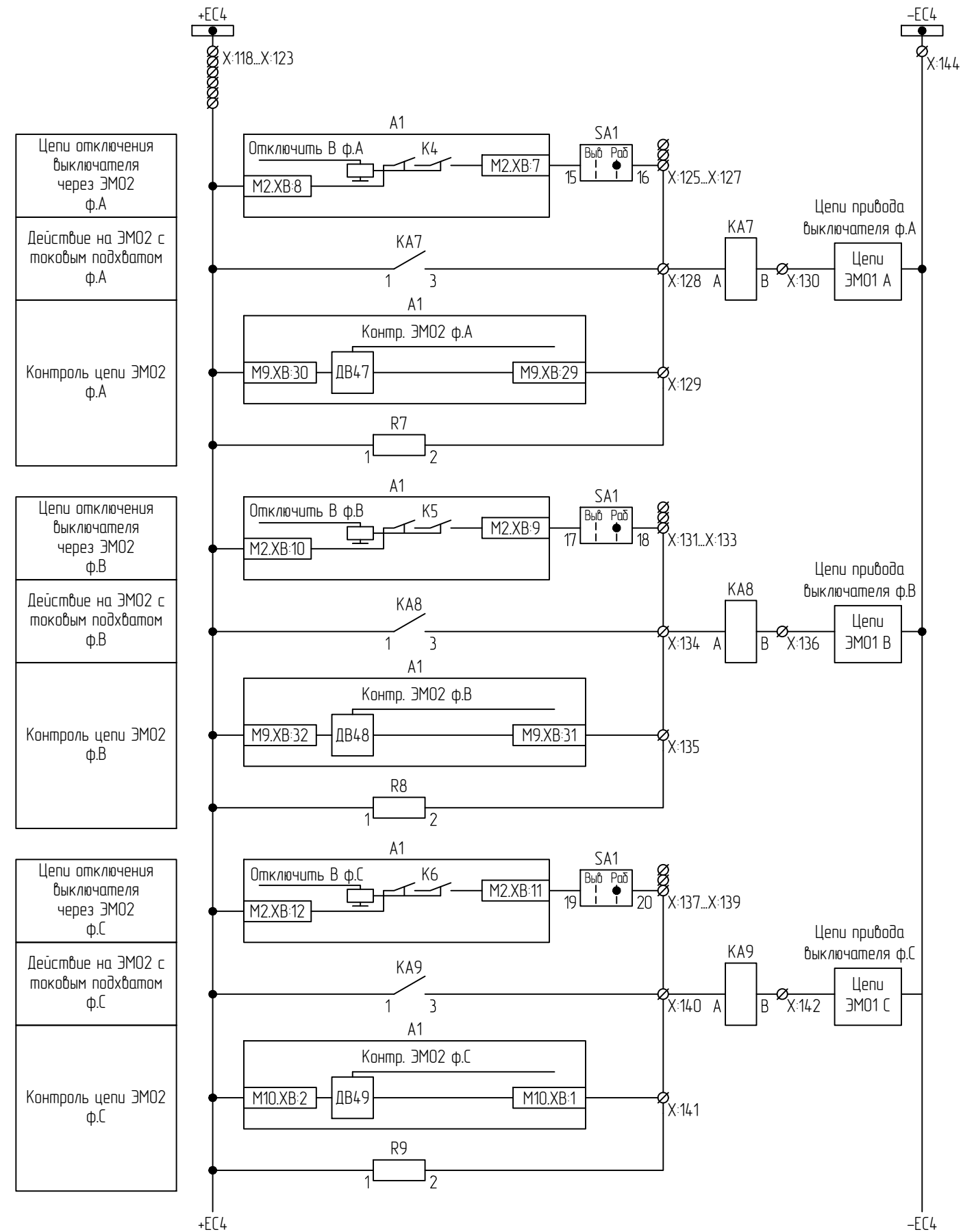
Цепи ЭМ02
