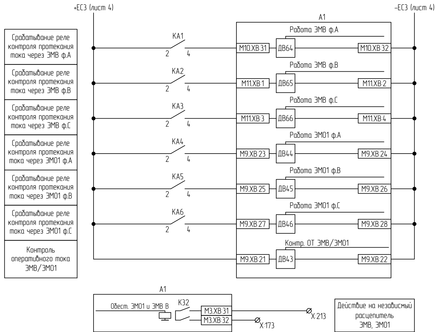
Цепи ЭМВ/ЭМ01
